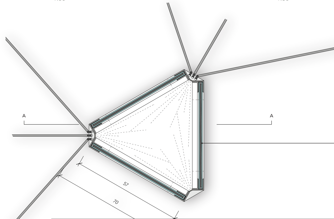
Grunnmynd 1:20
